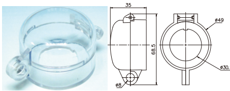
TN3-GR 圓形護蓋
